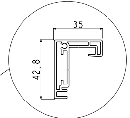
Perfil guía zip Guide profile zip
