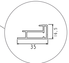
Tapa perfil guía zip Front zip guide profile
